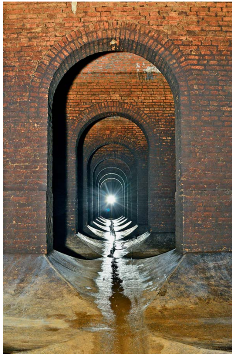
▲ Společný žlab. První vodojem je rozdělen na devět rovnoběžných oddílů navzájem propojených odtokovým žlabem.
